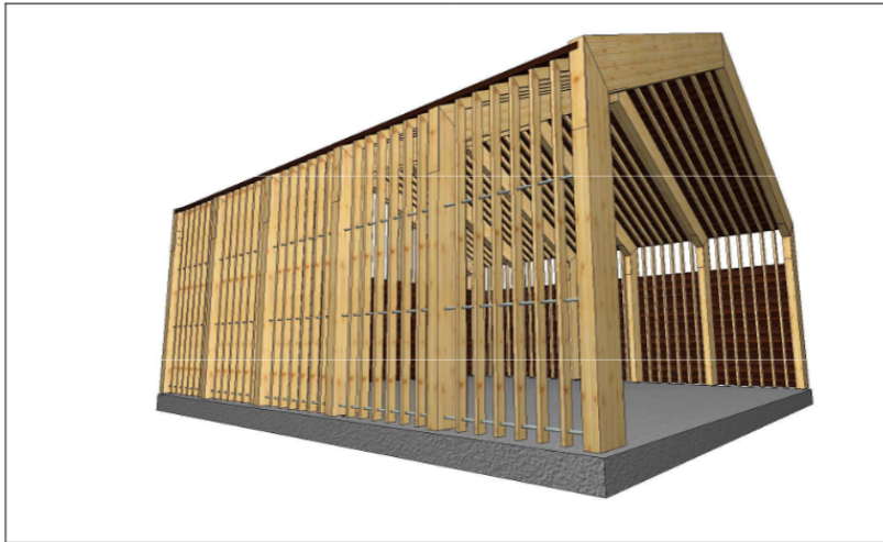
Skizze der Firma Foffa Conrad Holzbau AG für den Unterstand
